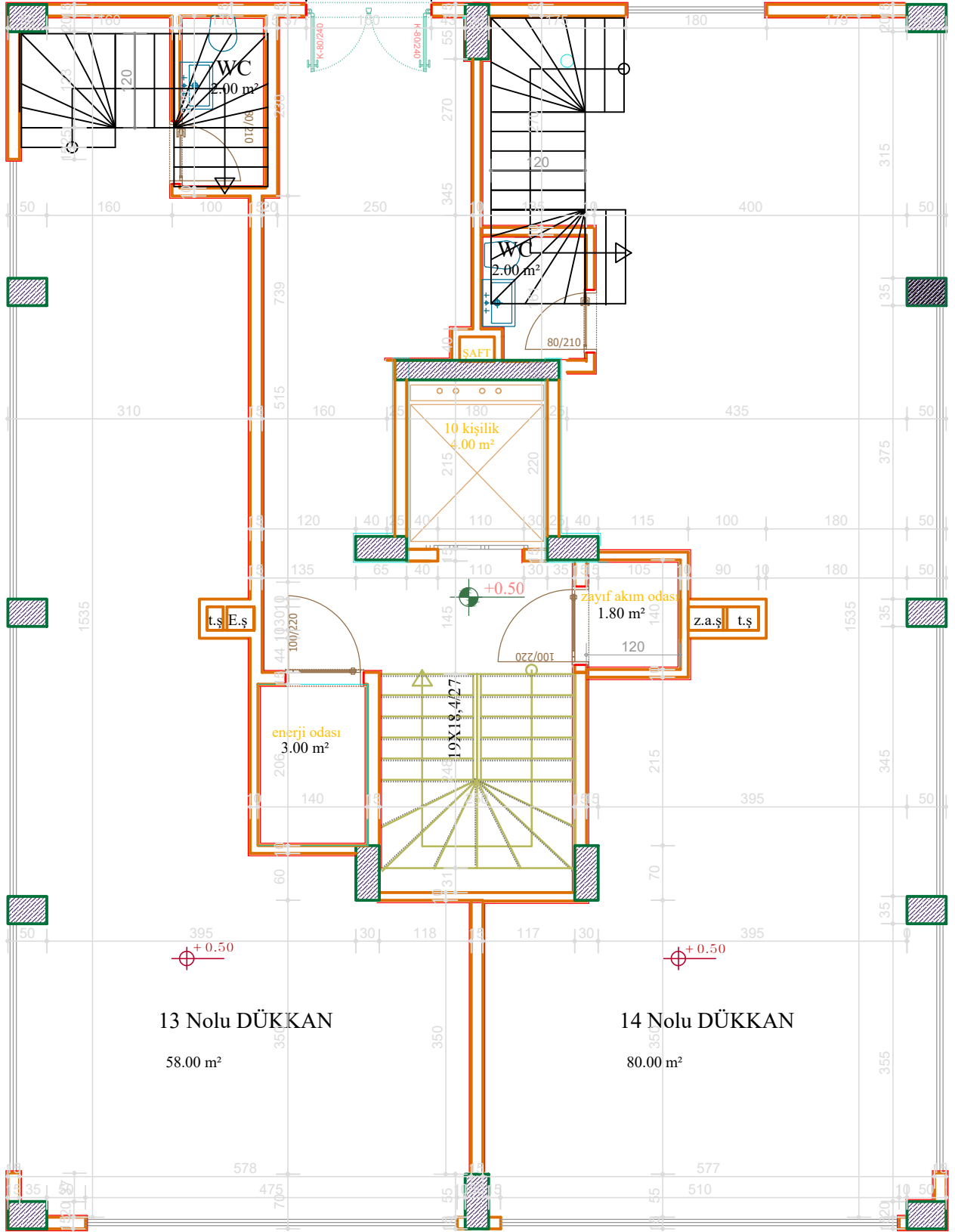
ZEMİN KAT PLANI ÖLÇEK : 1 / 50
